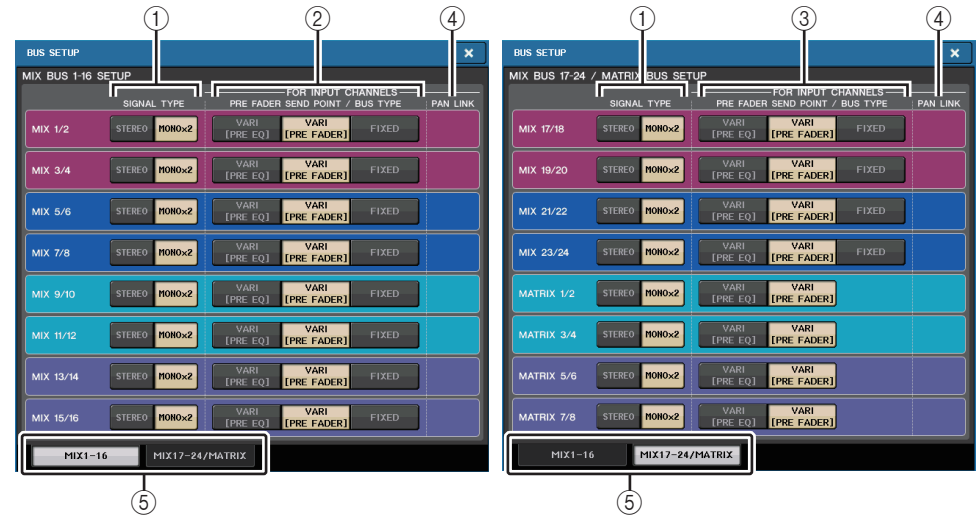
Страница MIX 1–16
