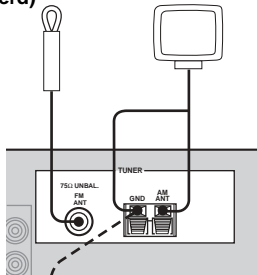
FM binnenantenne (meegeleverd) AM ringantenne (meegeleverd)
