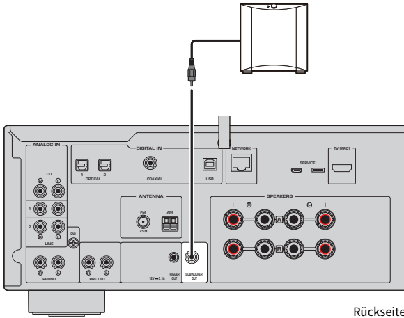
Subwoofer (mit integriertem Verstärker)
